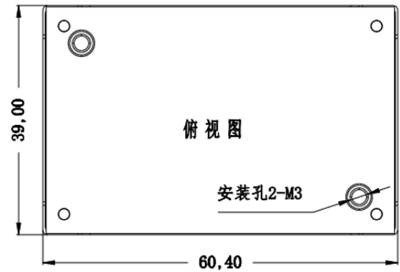
标准型 60.4*39*12.7mm
